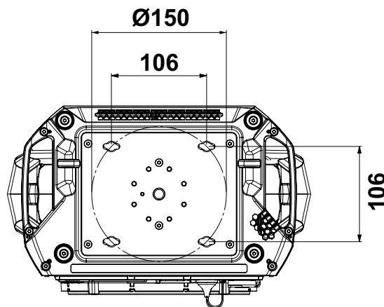
Figure 4: Points de montage des embases Oméga
